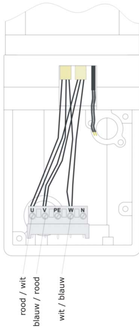
3x230 V
