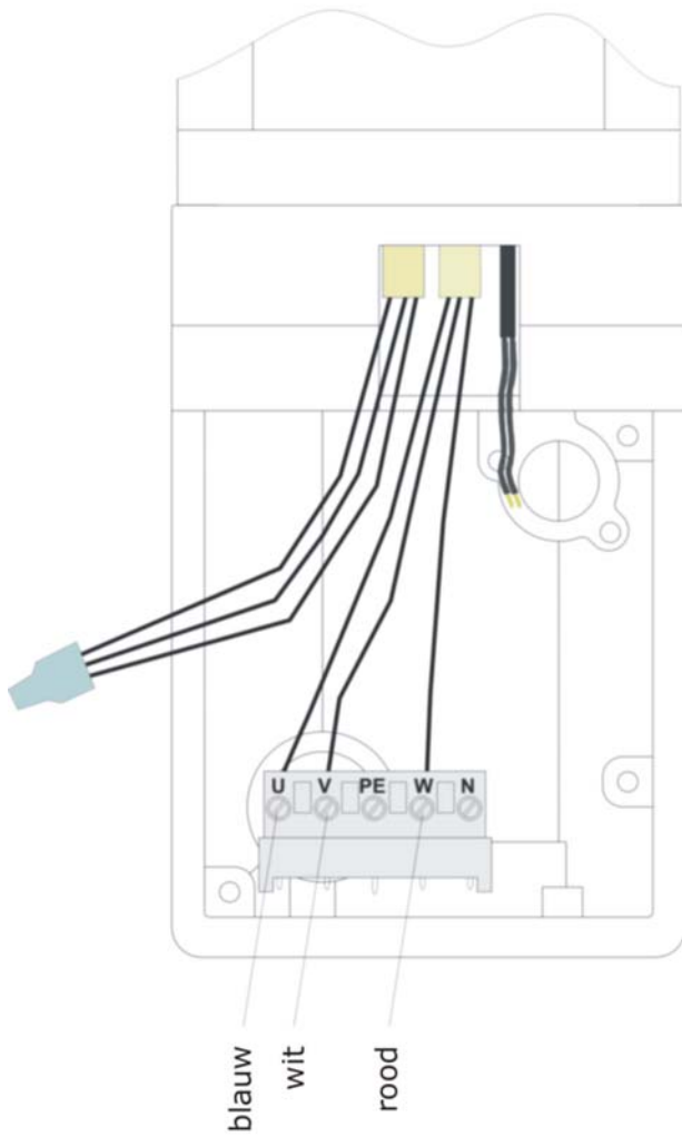
3x400 V
